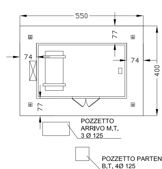
PLANIMETRIA SCALA 1:100
