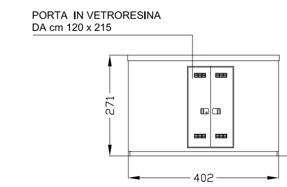
PROSPETTO FRONTALE SCALA 1:100
